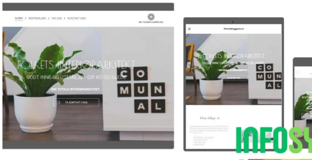
Nettsidebyggeren grafikk
